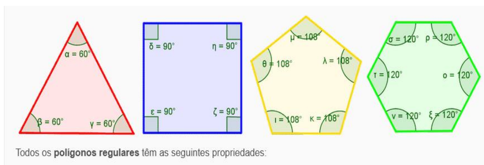
Figura 1: Polígonos regulares
